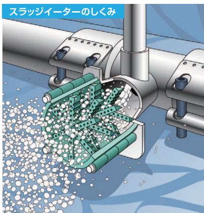
スラジイーターのしくみ
